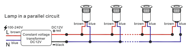
DC 12V input
