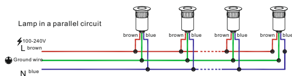
100-240V input
