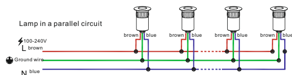
100-240V input
